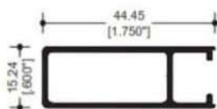
67821 CERCO PUERTA
