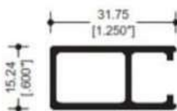
8320 CERCO VENTANA
