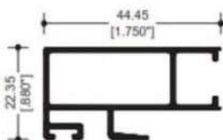
69955 TRASLAPE PUERTA
