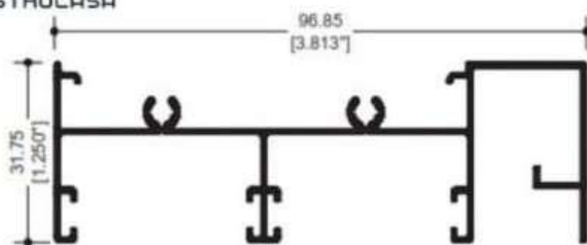
67862 CABEZAL MOSQUITERO COLGANTE
