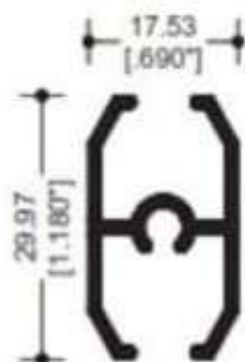
63728 PARA CUADRÍCULA RECERCADO 2"
