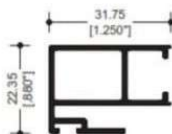
39954 TRASLAPE VENTANA
