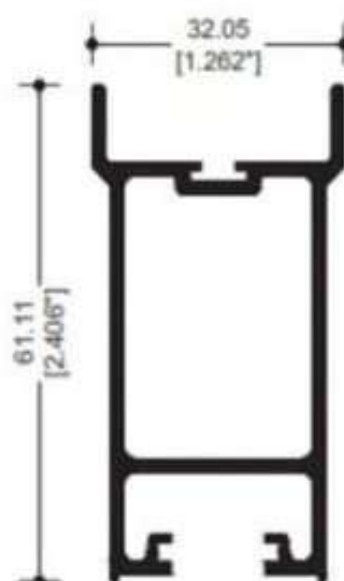
67850 CERCO OXXO
