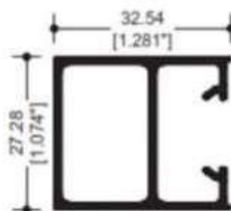
67843 CERCO VENTANA
