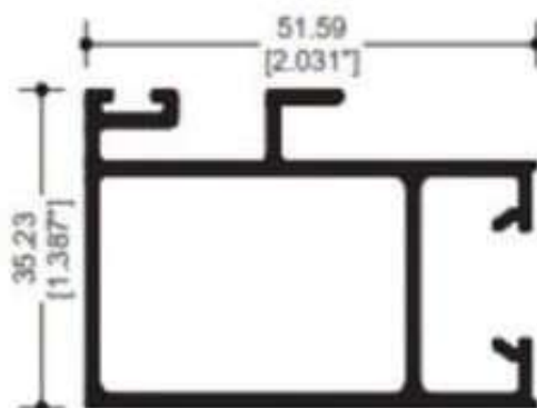
67848 TRASLAPE PUERTA
