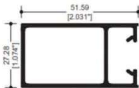
67847 CERCO CHAPA PUERTA
