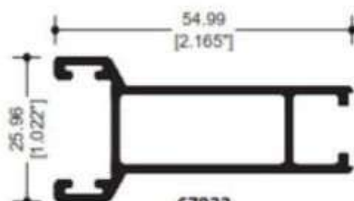
67822 CERCO OXXO PUERTA
